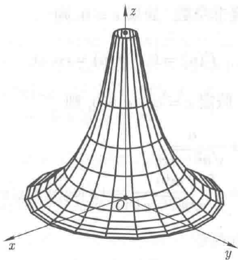
图 1: 伪球面
